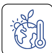
Changement climatique
