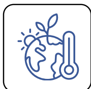
Changement climatique
