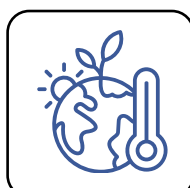
Changement climatique
