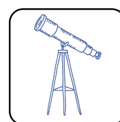
Astronomie
